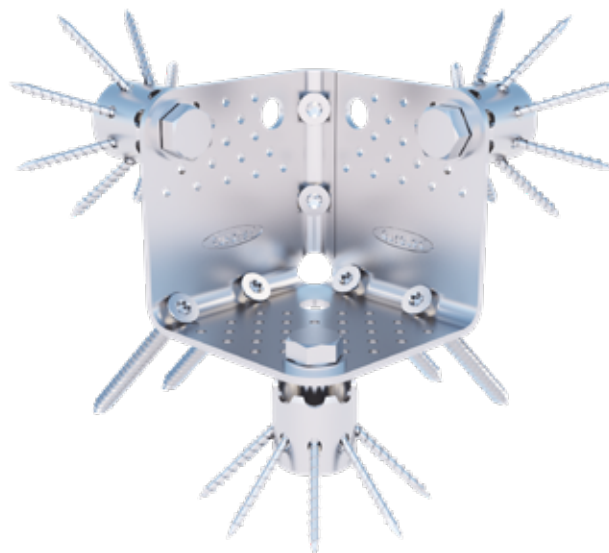
Systeminnenecke CLT mit IdeeFix
