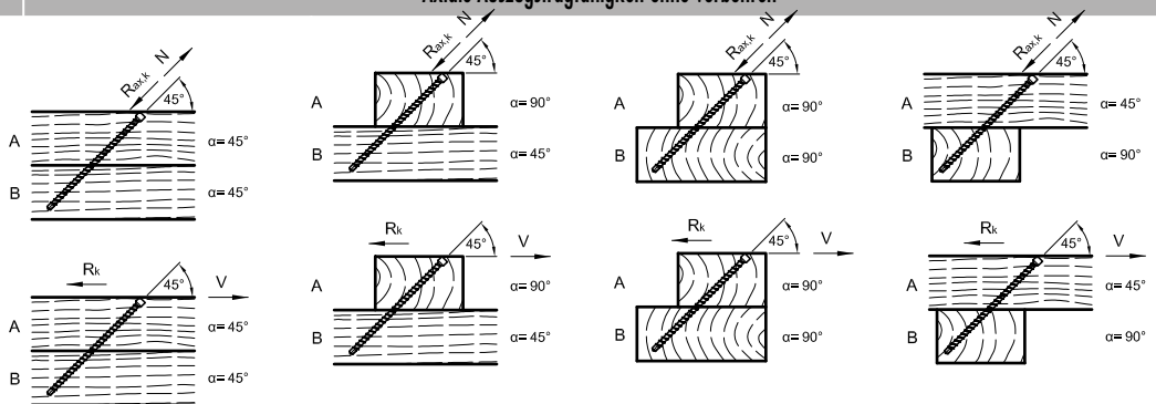
Charakteristischer Wert der Tragfähigkeit der Verbindung R_k nach ETA-11/0024
