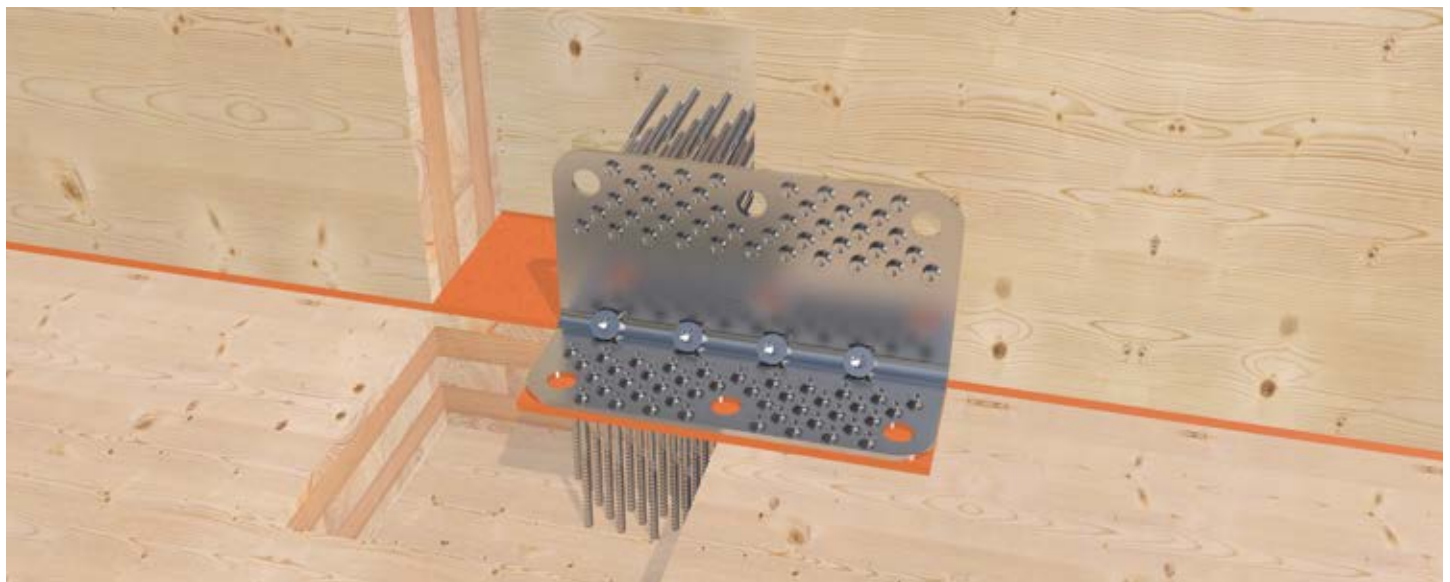
Systemwinkel CLT zur Befestigung einer Wand am Holzfußboden des Obergeschosses.
